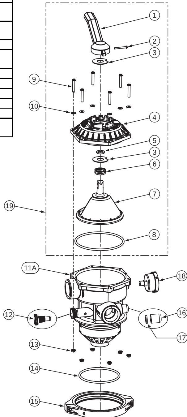
VALVULA ESTILO DE ABRAZADERA
