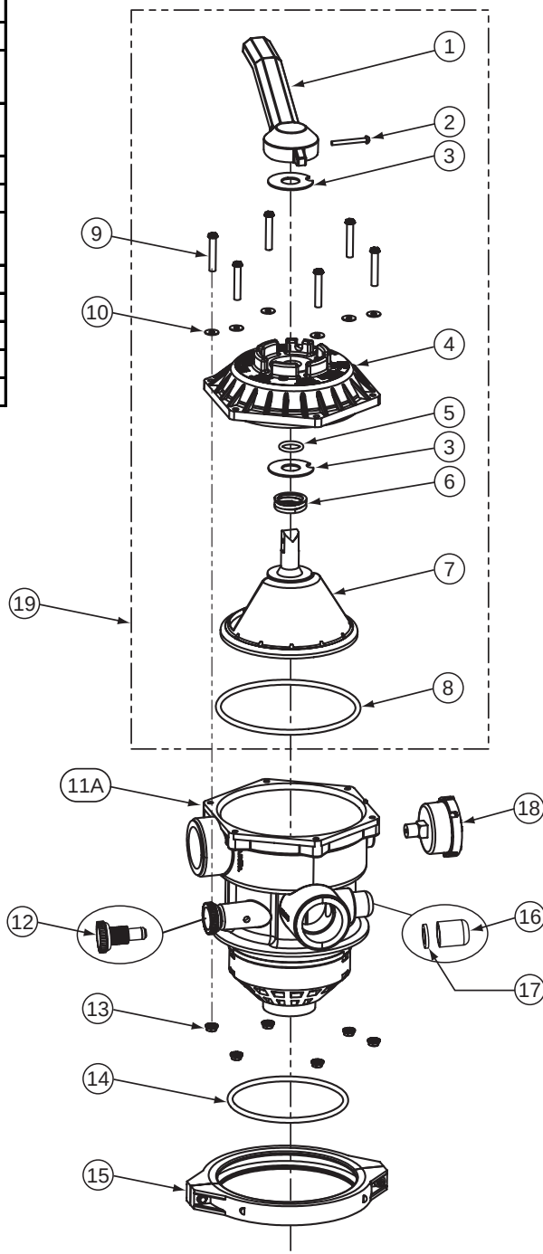
VANNE A FIXATION PAR COLLIER
