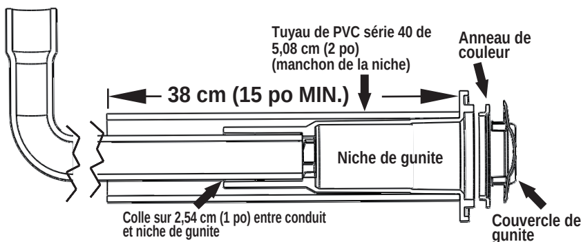
Option 2 : Du conduit à la lumière – Schéma d'installation
