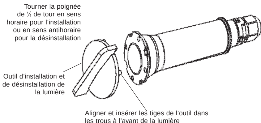
Outil d'installation et de désinstallation de la lumière colorée GloBrite®
